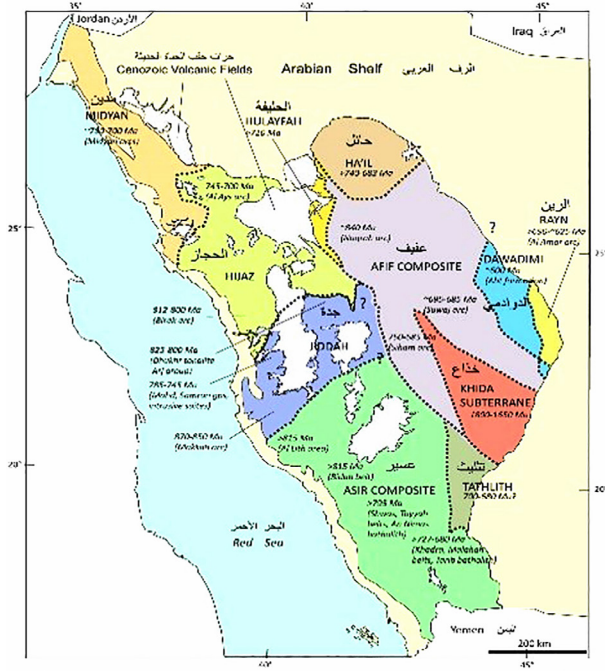
موقع إقليم حائل الجيولوجي ضمن الدرع العربي في وسط شمال المملكة.
